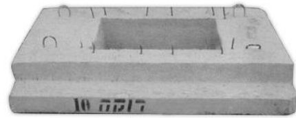
תקרה לתא תקשורת A2 פתח מרובע מידות התקרה 163/111/20
